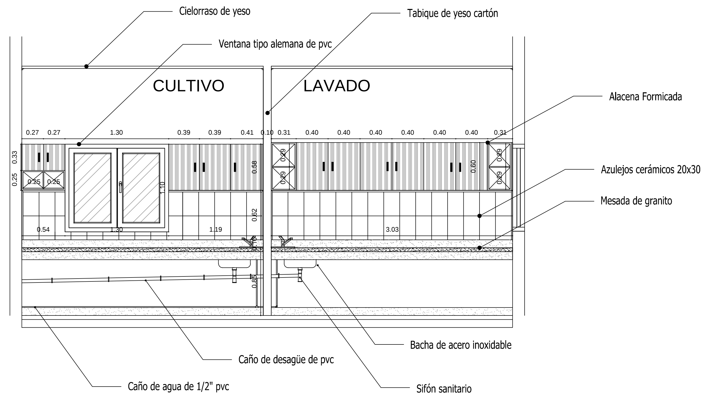
CORTE A-A'
