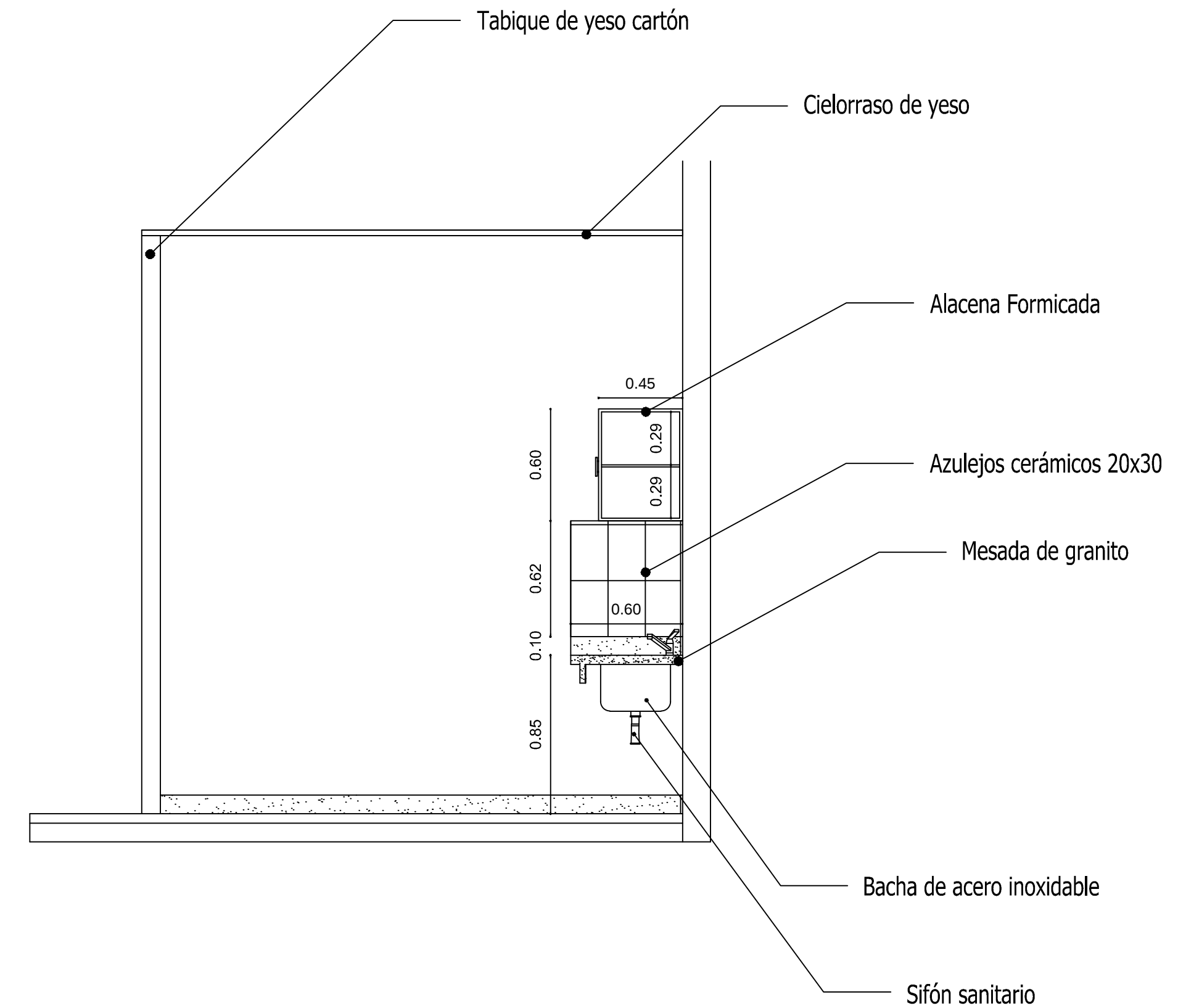
CORTE B-B'
